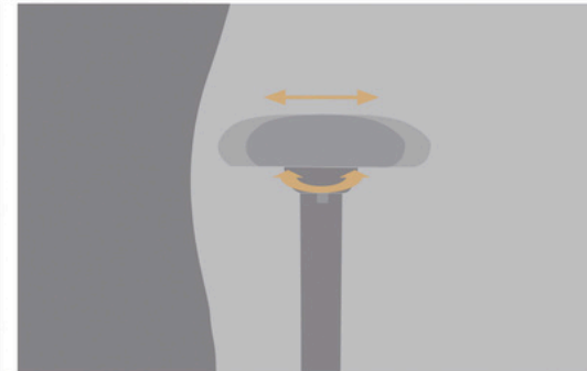
Kolçak sağa-sola ve açı ayarı: 30 mm Açı ayar aralığı: -20° / +25°
